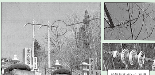
設備被害:がいし破損
